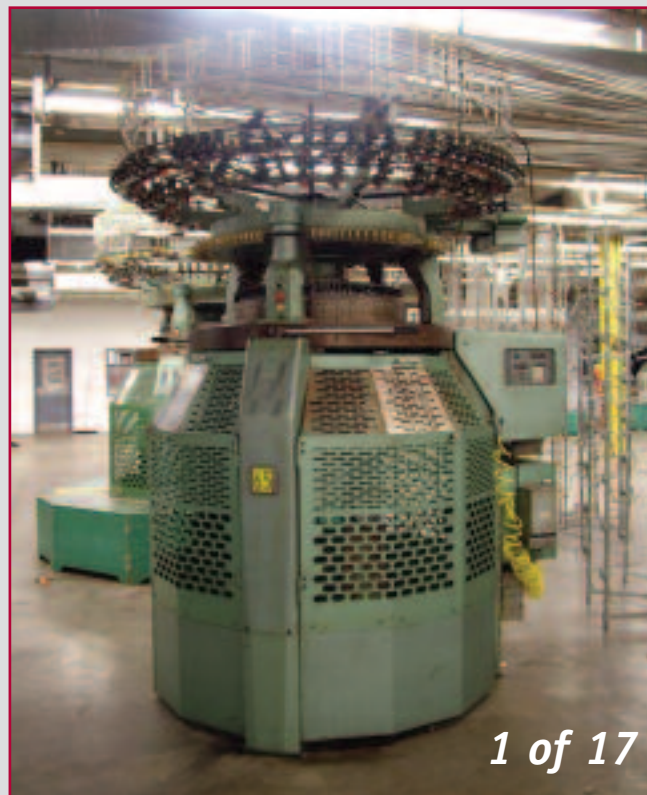
MONARCH FIL-8AE
